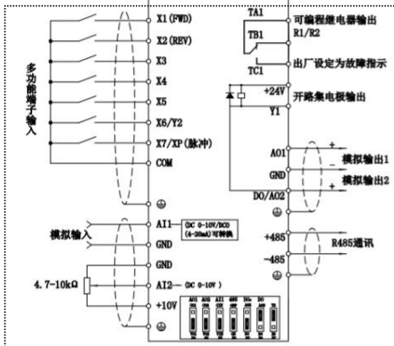
控制回路
