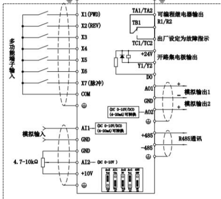
控制回路
