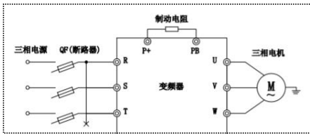
主回路
