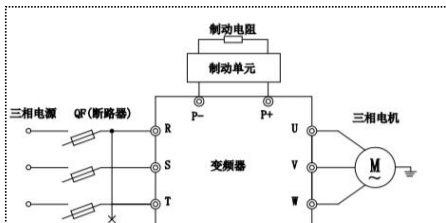
主回路
